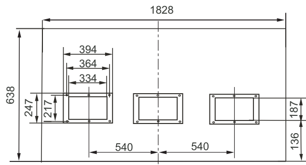
Схема расположения отверстий для болтов крепления воздуховода воздуховыпускного отверстия GC-DH192HWN1
